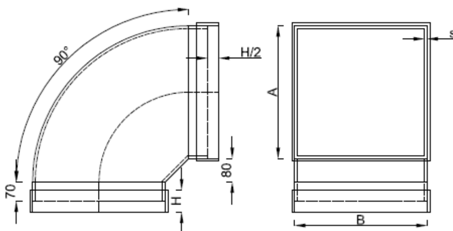
TAB1. Wymiary główne i grubość ścianek kolan i łuków prostokątnych z materiału PP / PPs
