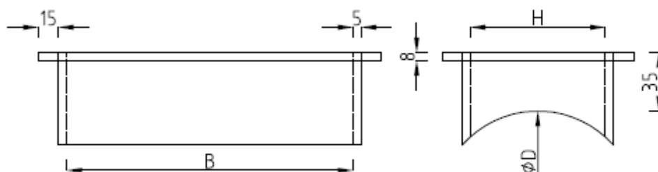
TAB1. Wymiary główne i grubość ścianek sztuczerów prostokątnych z materiału PP / PPs
