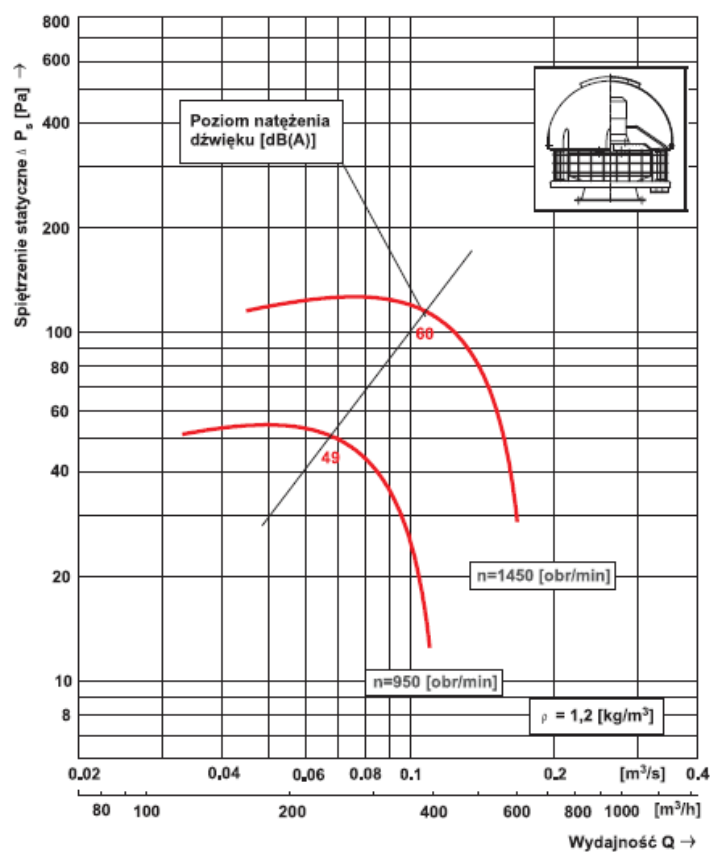
Charakterystyka przepływowa wentylatora dachowego WDc/s 16
